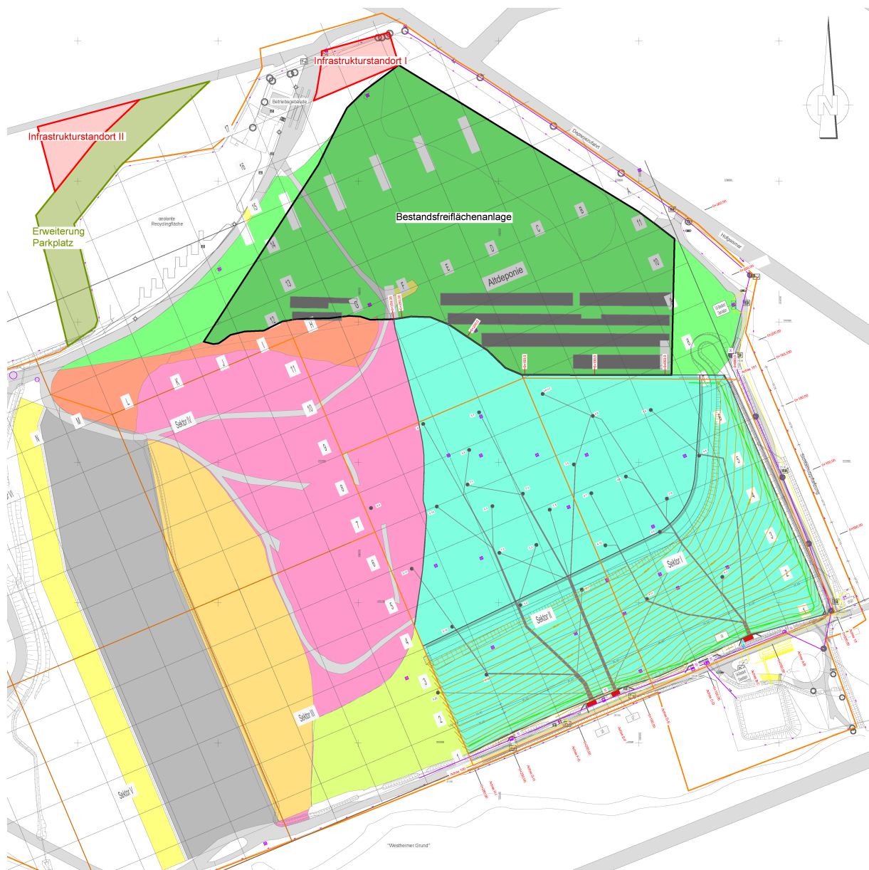
Abbildung 1: Bestandslageplan Deponie Kirschenplantage, Stand 09/24 (Quelle: SIG-Hessen Ingenieure, ohne Maßstab)
