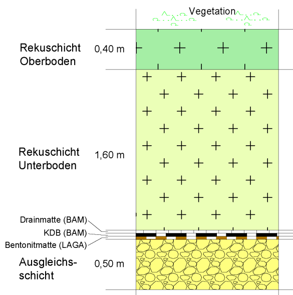
Abbildung 14: Detail Aufbau Oberflächenabdichtungssystem (Quelle: SIG-Hessen Ingenieure, ohne Maßstab)
