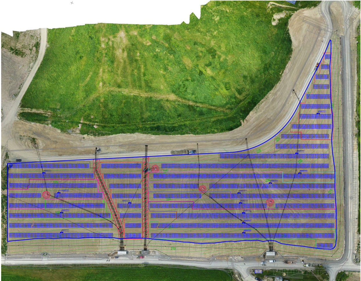
Abbildung 12: Lageplan Bauabschnitt 1 (BA1) der PV-Freiflächenanlage inklusive Darstellung des Entgasungssystems, ohne Maßstab, nicht genordet (Quelle: SIG-Hessen Ingenieure)
