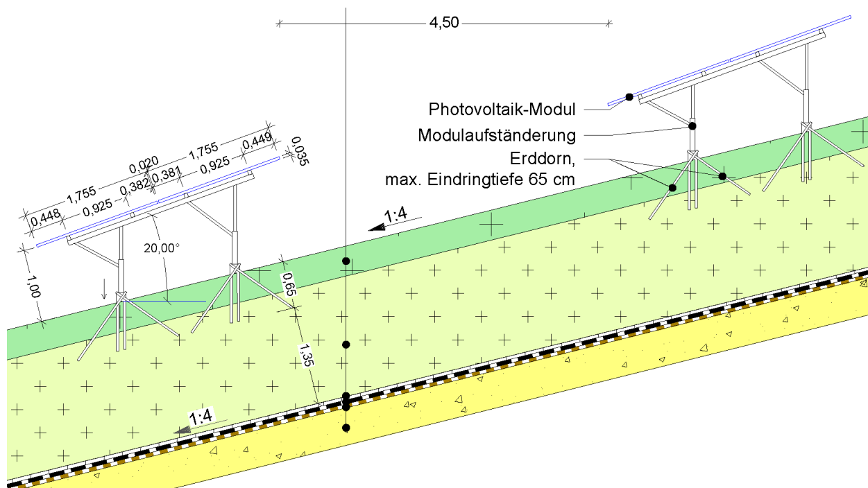
Abbildung 13: Detailplan Modultisch und Gründung (Quelle: SIG-Hessen Ingenieure, ohne Maßstab)
