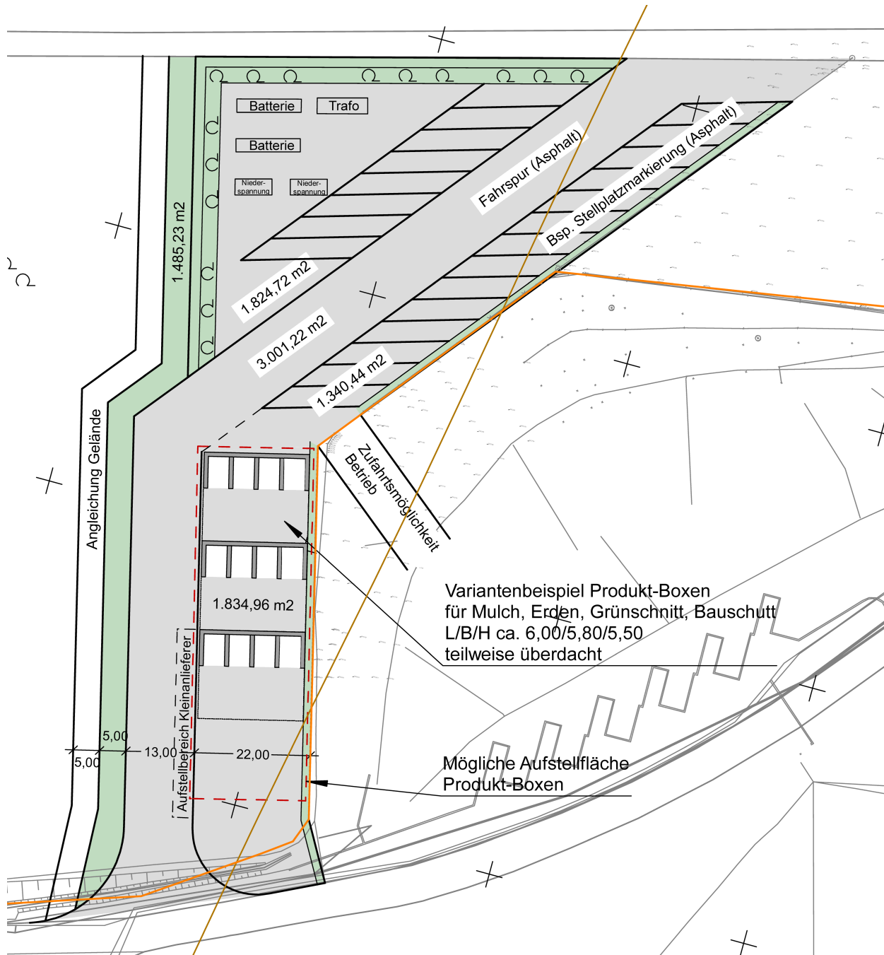
Abbildung 11: Lageplan Infrastrukturangebot (ohne Maßstab, Quelle: SIG-Hessen Ingenieure)
